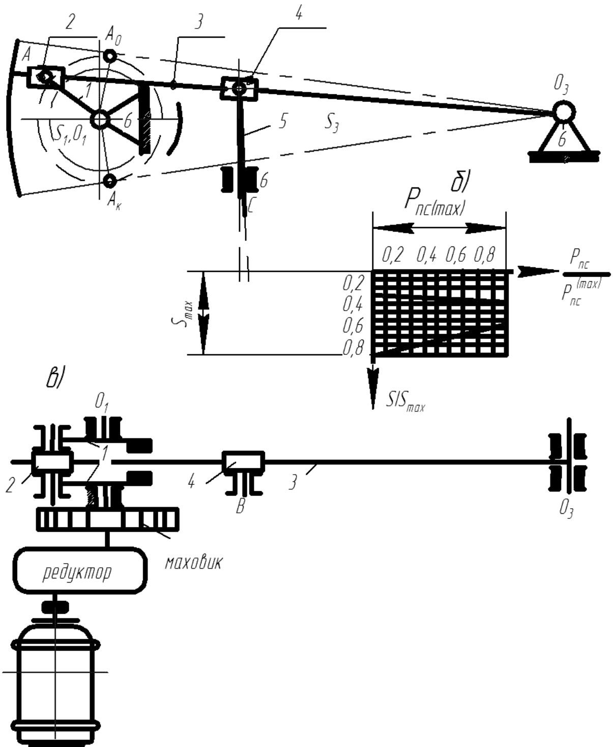
а - схема рычажного механизма пресса; б - механическая характеристика шивного пресса; в - схема машинного агрегата.
