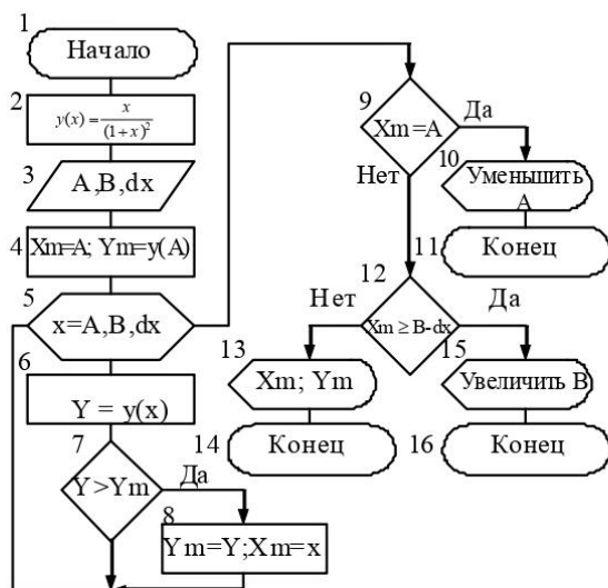
Схема алгоритма
