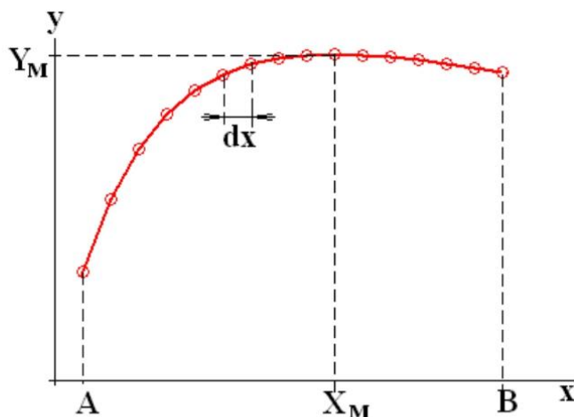
Схема алгоритма
