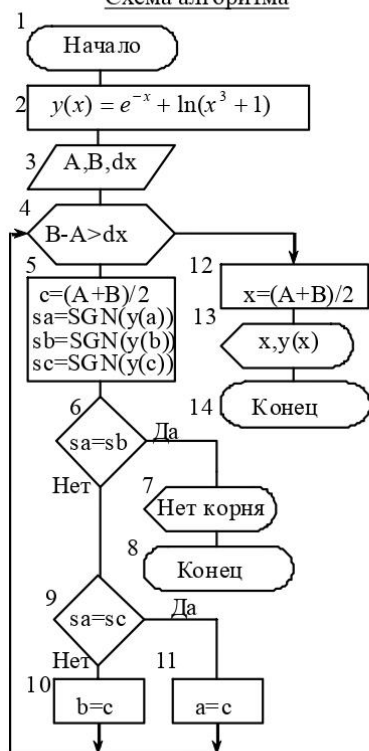
Схема алгоритма
